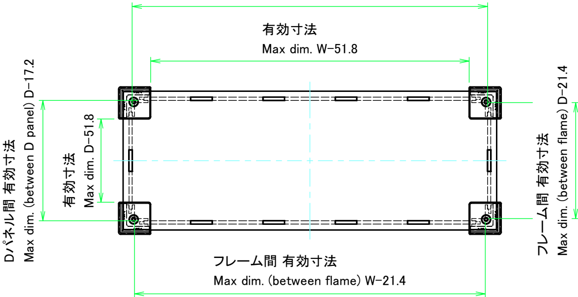
Dパネル1 / D Panel 1
