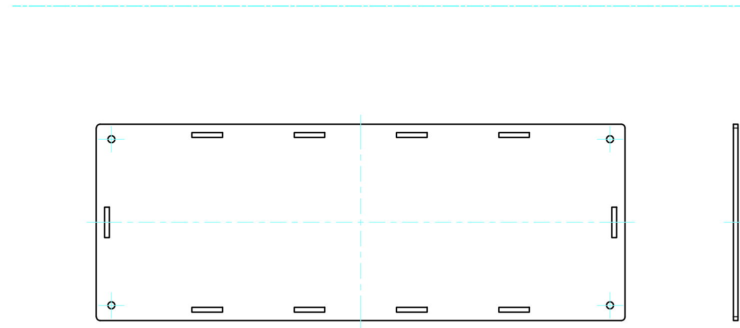
上カバー表面 / Top cover Frontside
